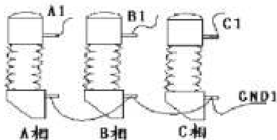
图 6 断口接线图
