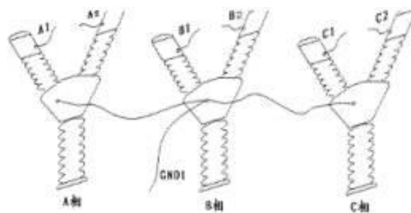
图 7 断口接线图
